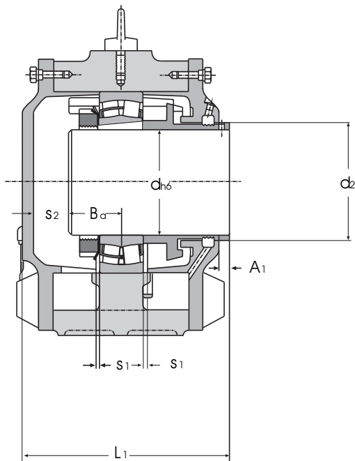
Ausführung AL
