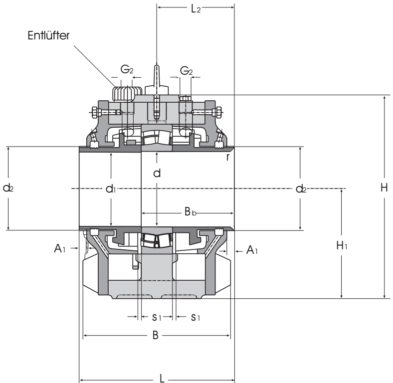
Ausführung BF
