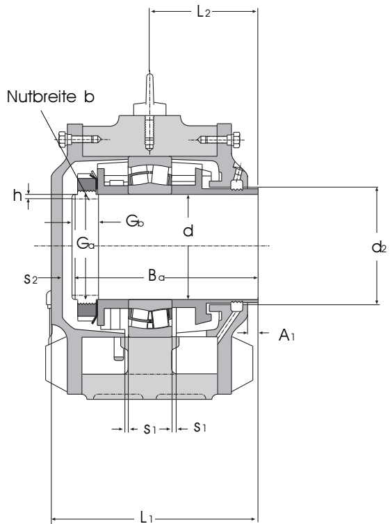
Ausführung AF
