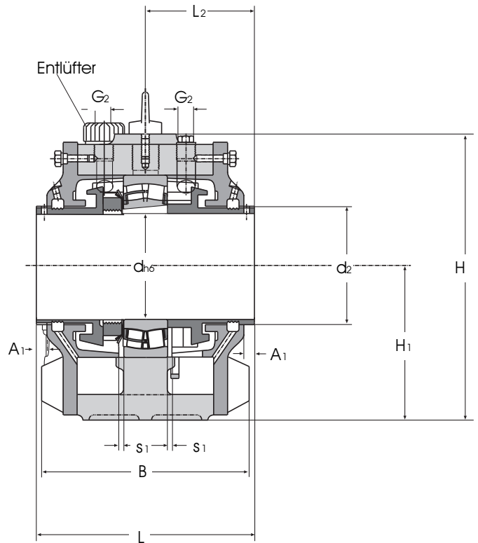
Ausführung BF
